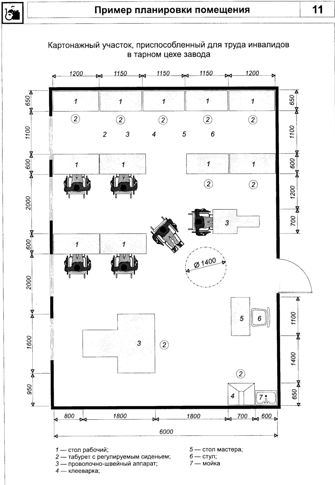
"Рис. 11. Пример планировки помещения"
