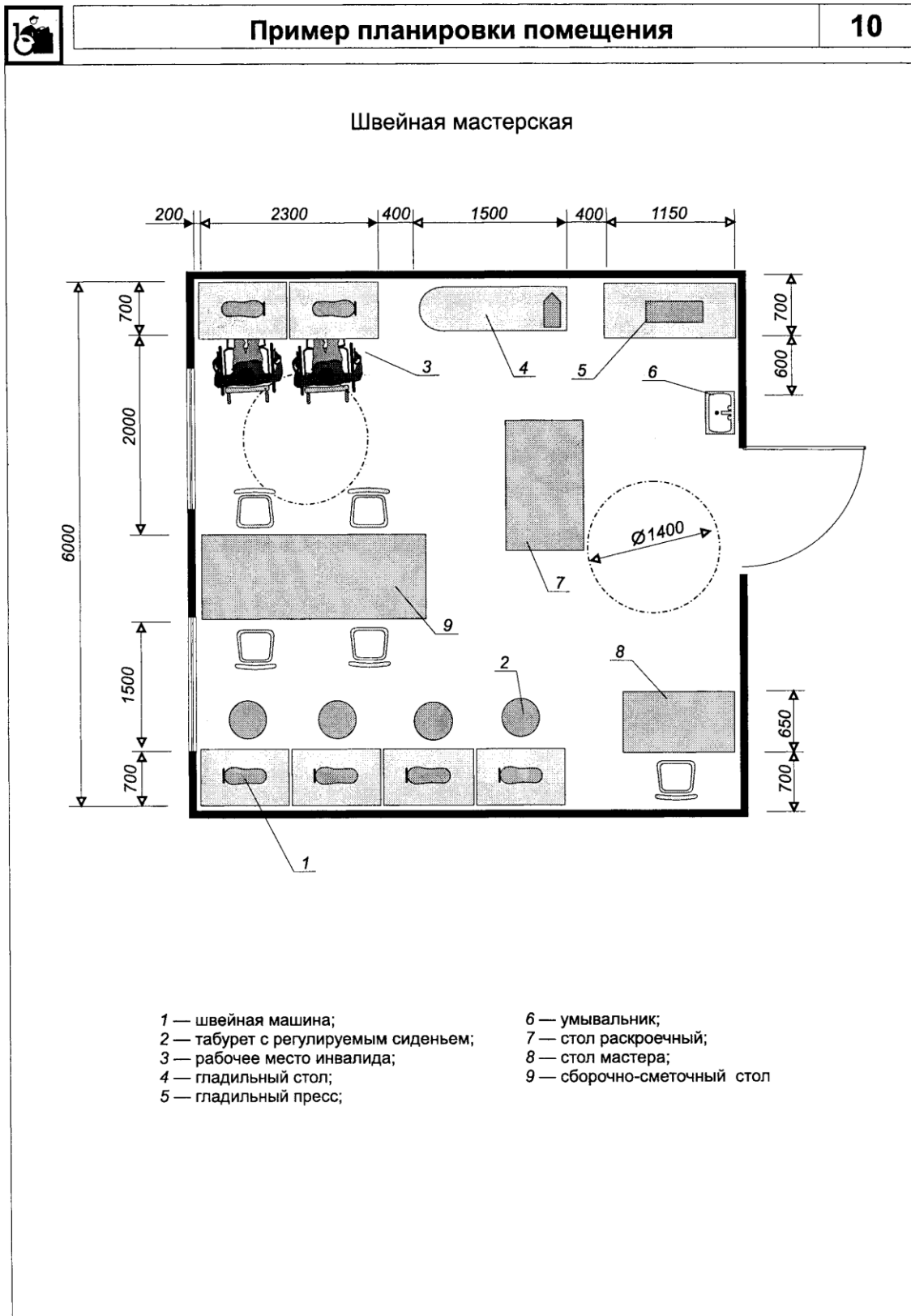
"Рис. 10. Пример планировки помещения"
