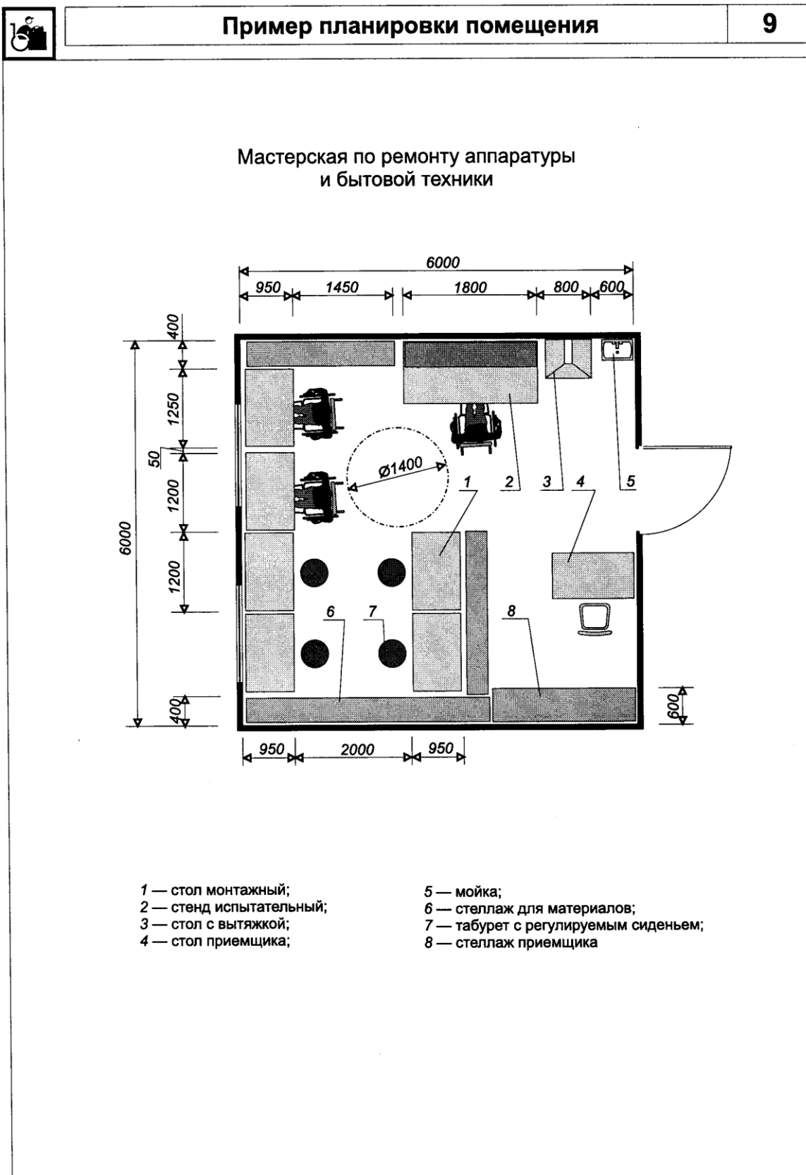
"Рис. 9. Пример планировки помещения"
