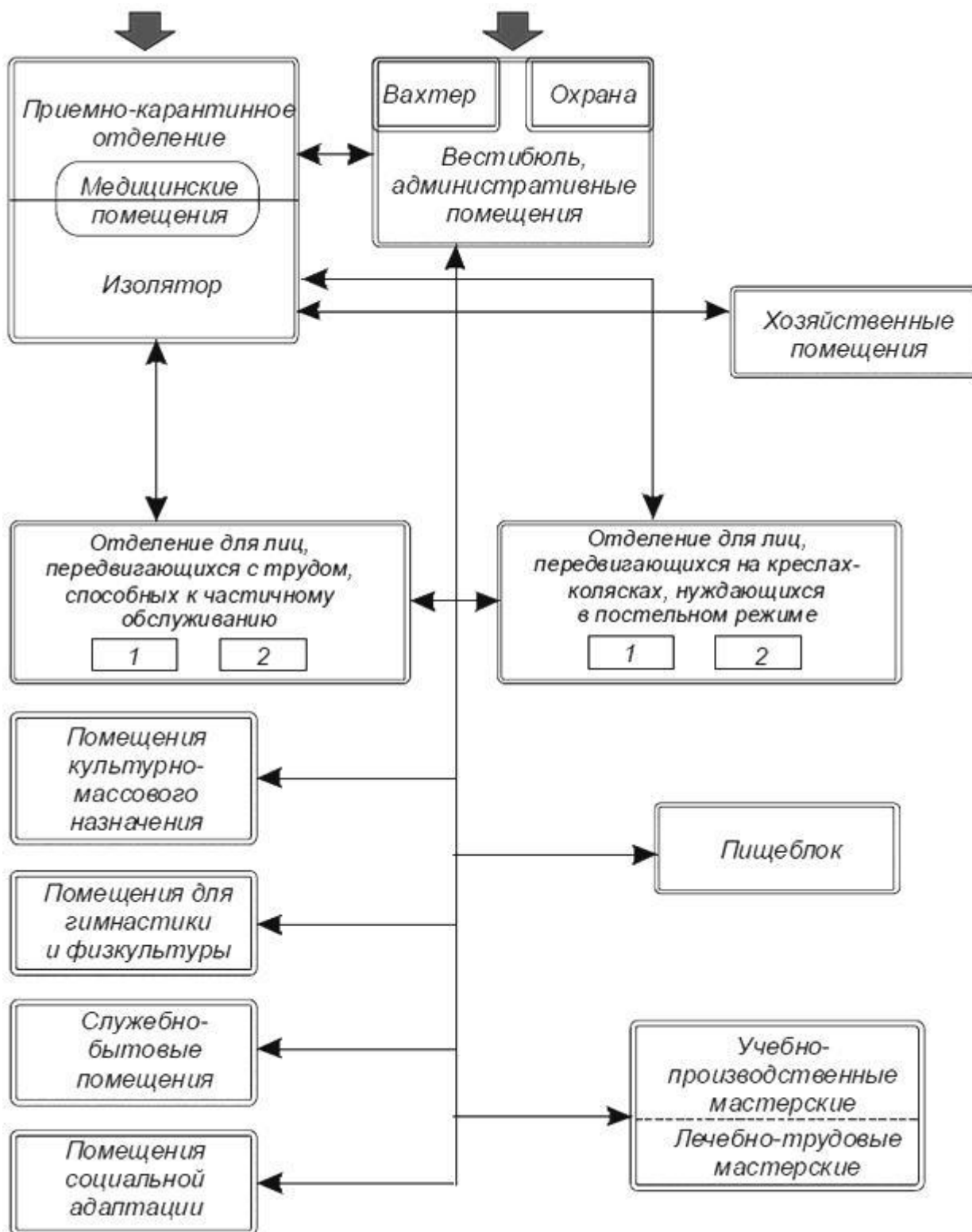
Рисунок Б.2 - Схема взаимосвязей жилых групп и помещения психоневрологического дома-интерната
