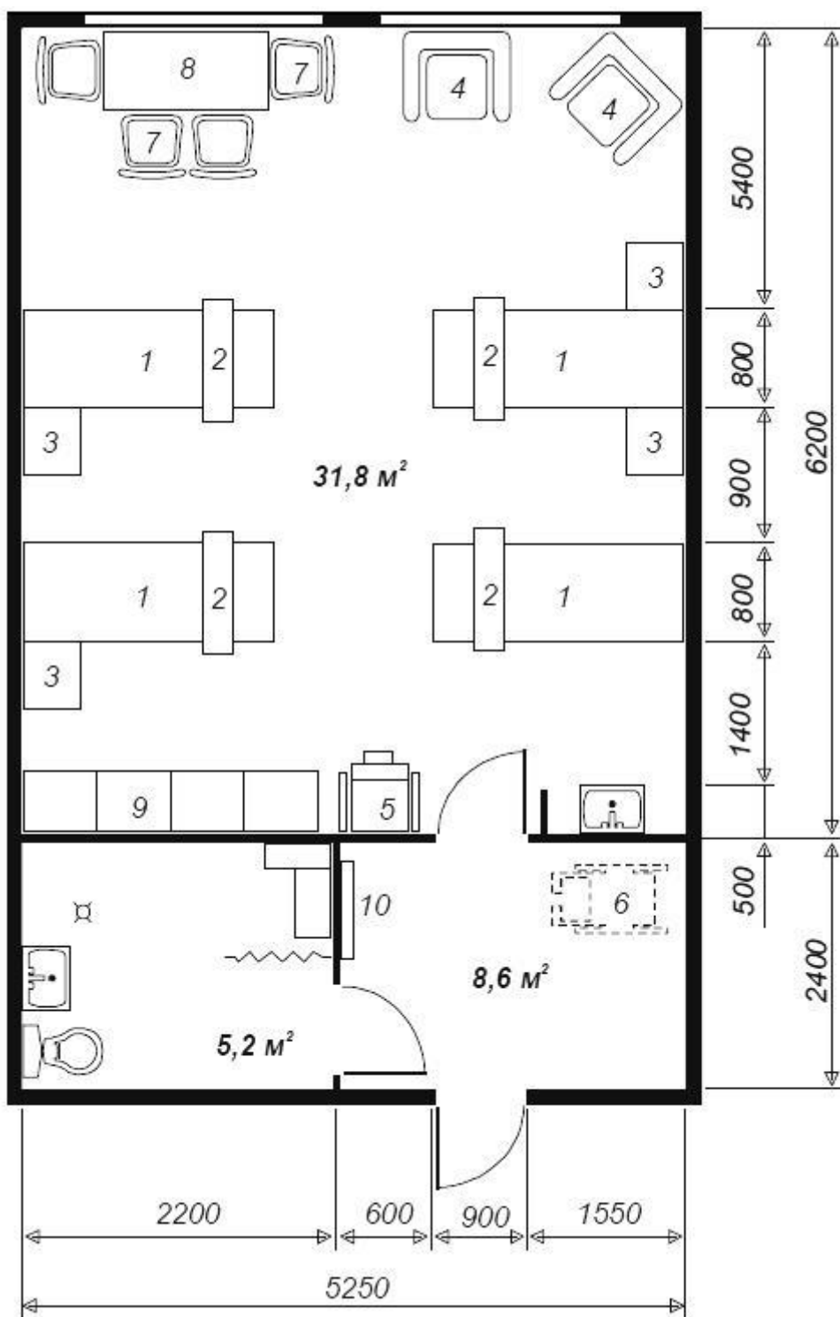
Рисунок Б.6 - Планировочная схема жилой ячейки ЖЯ-5
