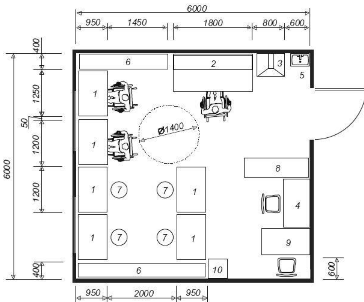
Рисунок Б.15 - Мастерская по ремонту аппаратуры и бытовой техники
