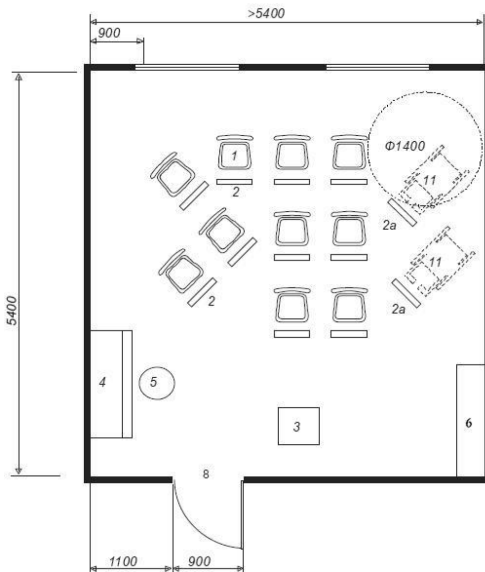
Рисунок Б.12 - Помещения для музыкальных занятий
