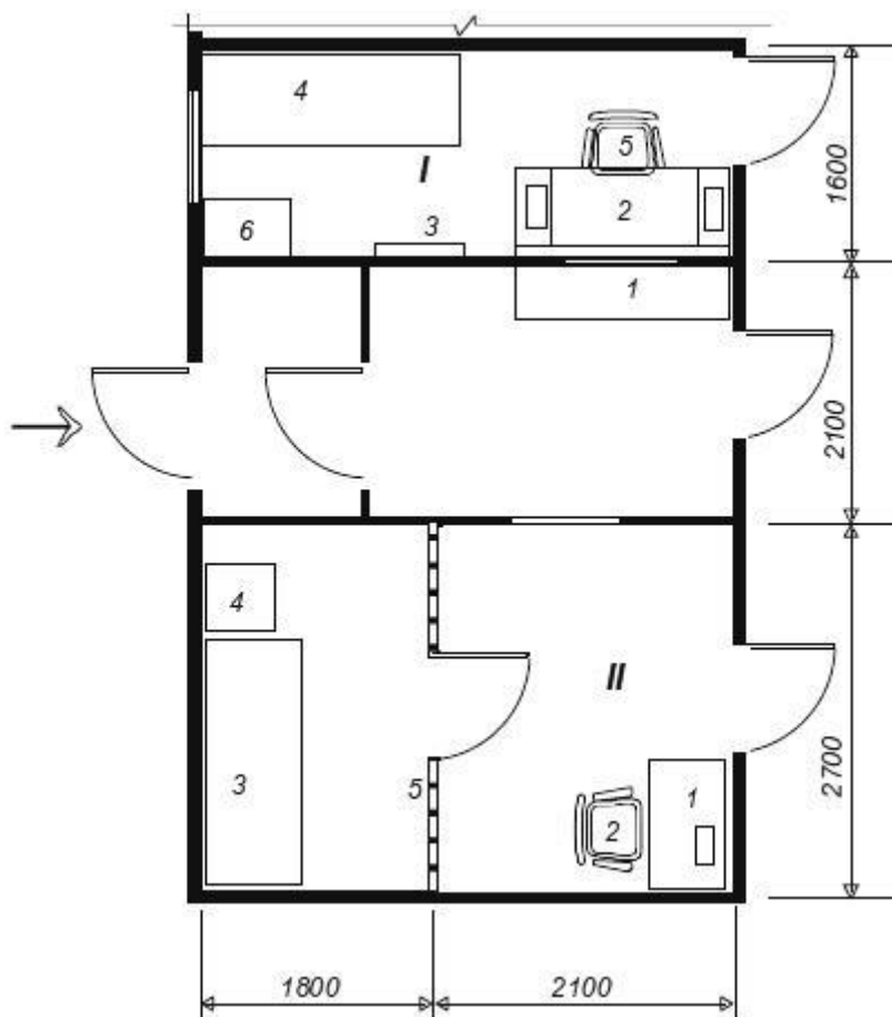
Рисунок Б.3 - Помещение охраны и безопасности
