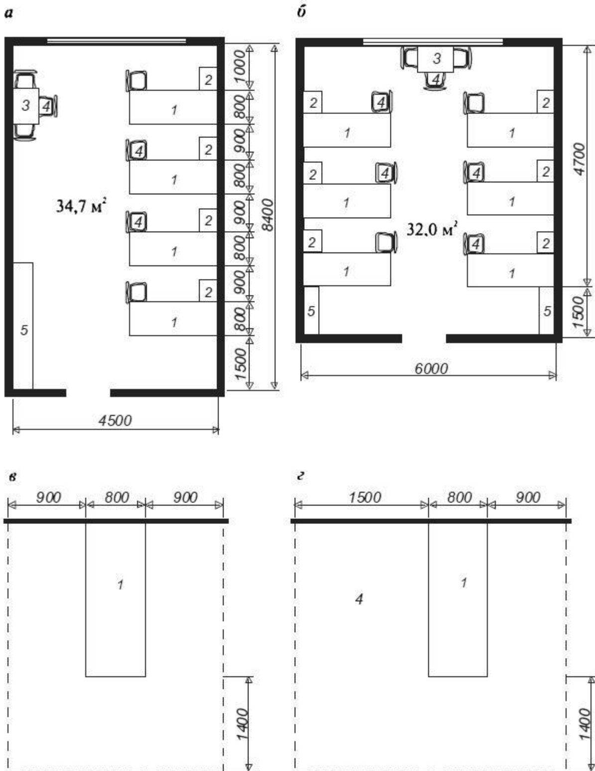
а - четырехместная жилая комната; б - шестиместная жилая комната; в - зона размещения кровати для лиц, способных к частичному самообслуживанию и передвигающихся по дому и прилегающему участку; г - зона размещения кровати для немощных лиц, передвигающихся в пределах жилой комнаты
