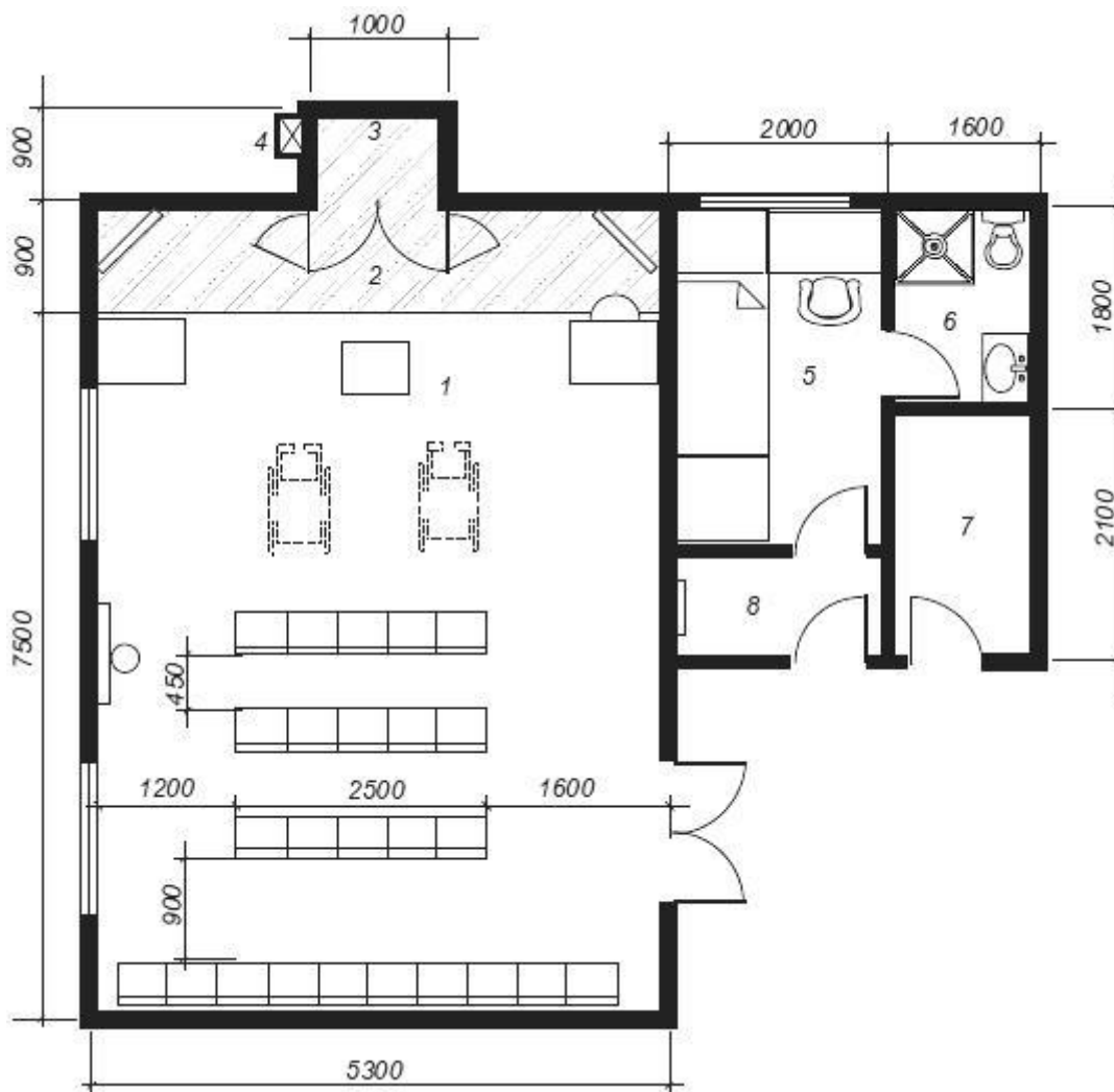
Рисунок Б.13 - Пример планировки зала для молитвенных собраний с подсобными помещениями
