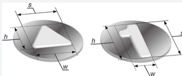
Рисунок 1 - Размер тактильного символа и тактильного знака
