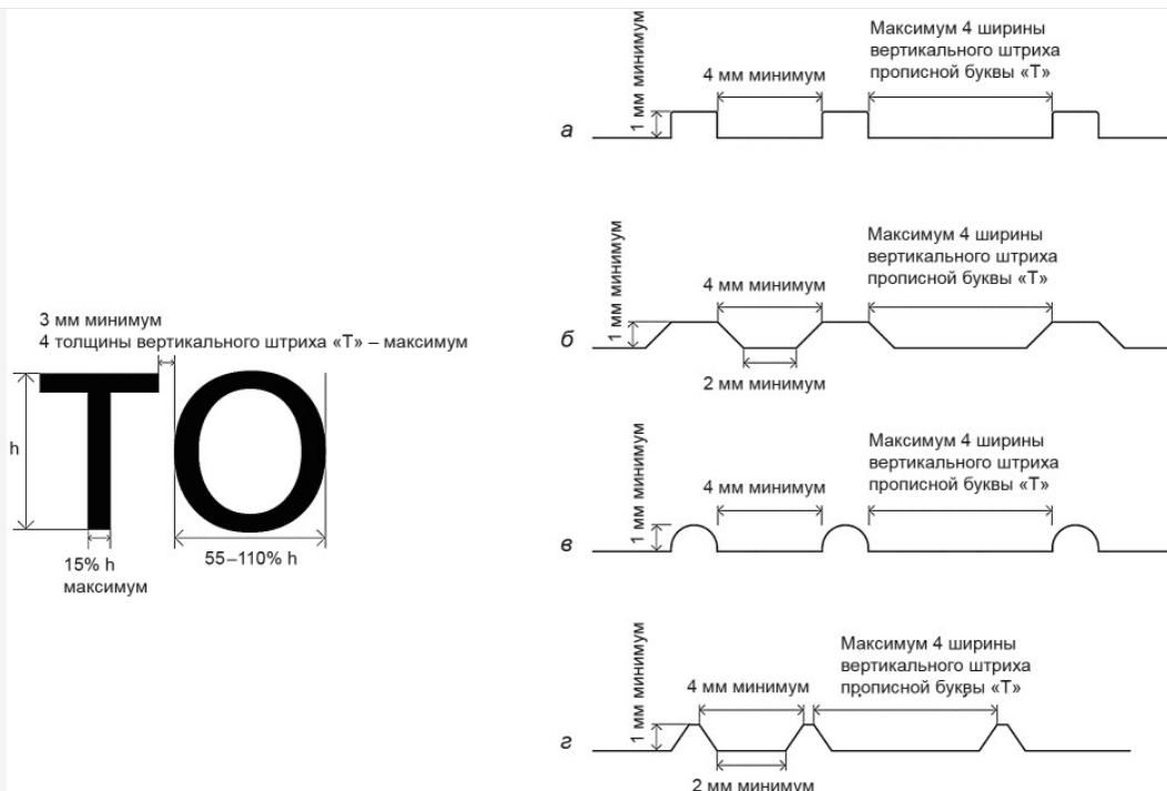
Рисунок 4 - Параметры шрифтовых знаков и рельефа (рифа) РЛШ
