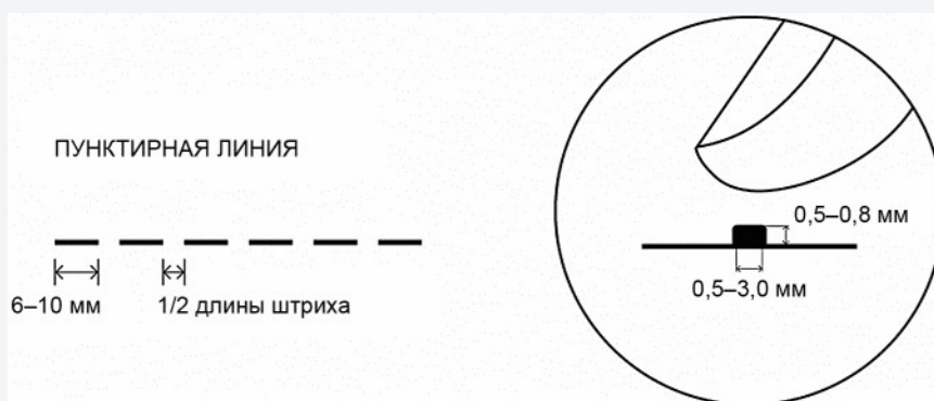
Рисунок 18 - Пунктирная линия
