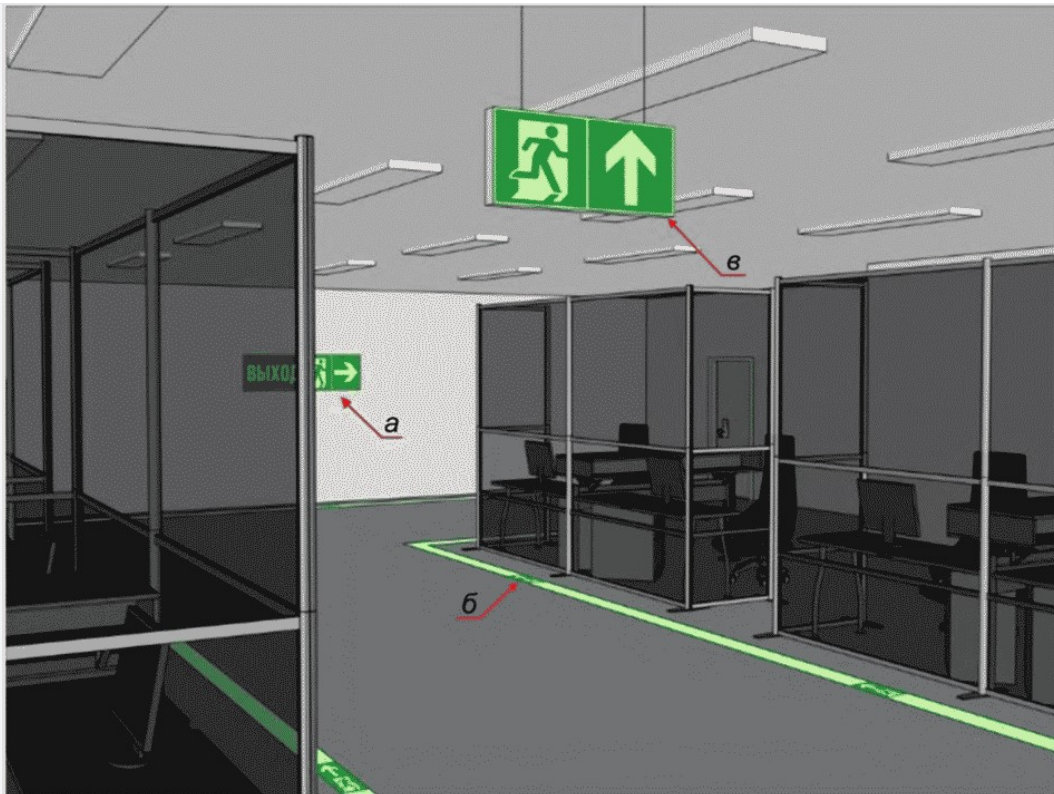
а - настенный комбинированный указатель направления эвакуации; б - напольная направляющая линия с включенным в ее состав указателем направления эвакуации; в - подвесной комбинированный указатель направления эвакуации Рисунок В.5 - Пример обозначения эвакуационного пути и направления эвакуации к выходу в помещениях со сложной конфигурацией размещения стеллажей, витрин, оборудования высотой более 1,5 м
